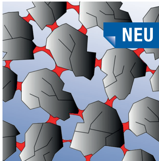
Gefüge mit der VITRA Hochleistungs-Niedrigbrandbindung
